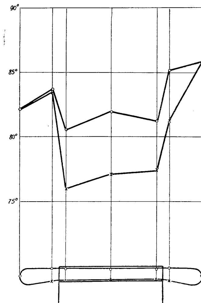
Рис. 1. Температурное поле двигателя АО2-42-4 при перегрузке. O — в верхней части паза, X — на дне паза.
