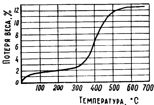
Рис. 1. Потеря веса
