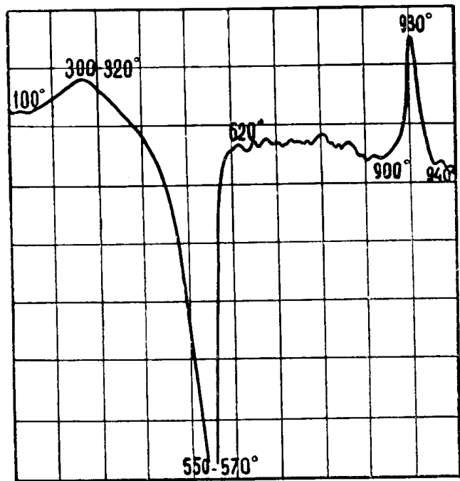
Рис. 2. Кривая ДТА
