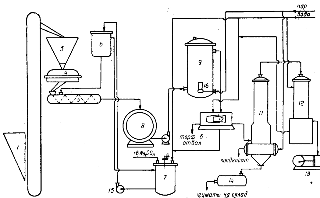
Рис. 1. Технологическая схема получения гуматов натрия: 1 — бункер для сырья, 2 — элеватор, 3 — промежуточный бункер, 4 — молотковая дробилка, 5 — шнек-смеситель, 6 — емкость для раствора, 7 — сборник, 8 — механический диспергатор, 9 — реактор, 10 — осадительная центрифуга, 11 — выпарной аппарат, 12 — поверхностный конденсатор, 13 — вакуумнасос, 14 — сборник гуматов, 15 — насос, 16 — эжектор
