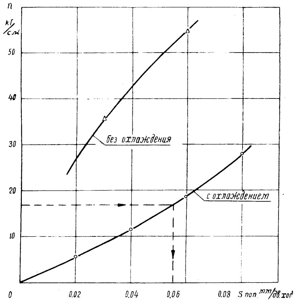
Рис. 3. Номограмма для выбора режимов шлифования
