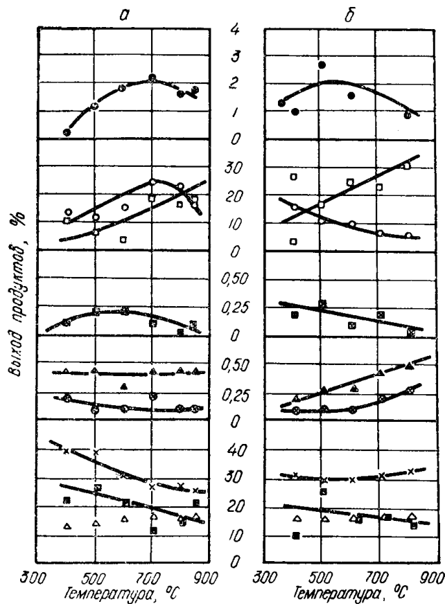
Рис. 1. Влияние температуры нагрева торфа и пиролиза летучих на выход химических продуктов. X — кокс, O — смола, □ — газ и потери, ● — газовый бензин, ■ — пирогенитическая вода, △ — углекислота, ▲ — аммиак, ⊕ — сероводород, ⊠ — непредельные углеводороды, а — без пиролиза, б — пиролиз летучих продуктов, чистый торф, степень разложения 15% (табл. 1)
