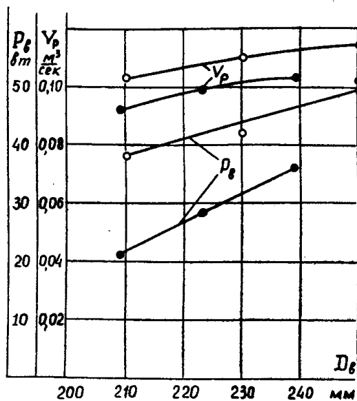
Рис. 2. Зависимость расхода воздуха V_p , вентиляционных потерь P_b от диаметра вентилятора D_2 :
