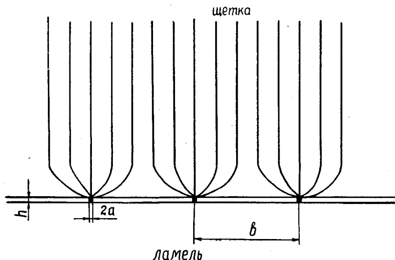
Рис. 1. Физическая модель скользящего контакта
