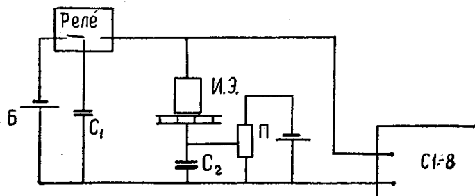
Рис. 5. Принципиальная схема измерительной установки для определения С
