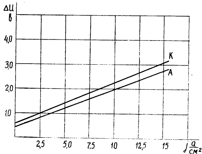
Рис. 7. Вольтамперные характеристики катодно- и анодно-поляризованной щеток поперечной цепи ЭМУ-12А
