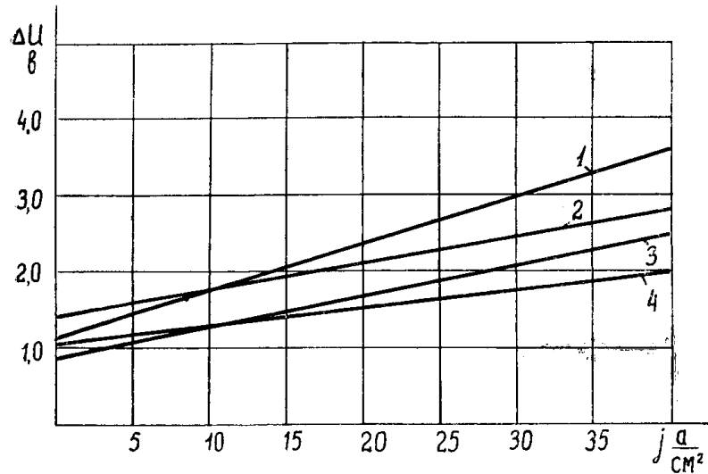
Рис. 6. Вольтамперные характеристики катодно- и анодно-поляризованной щеток продольной цепи ЭМУ-12А.
