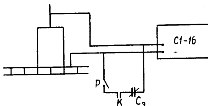
Рис. 4. Схема измерения максимального значения емкости
