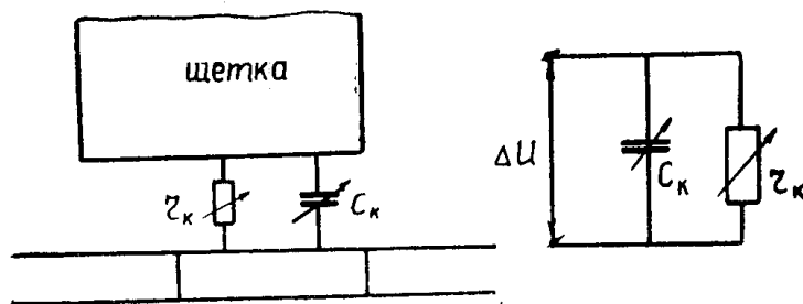
Рис. 2. Схема замещения скользящего контакта
