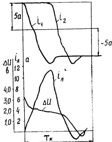
Рис. 3. Осциллограммы тока секций и падения напряжений.
