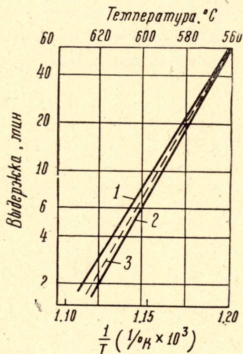
Рис. 1. Зависимость продолжительности выдержек эквивалентных отпусков от их температуры для стали Р18: 1 — закаленной от 1230°C; 2 — 1300°C; 3 — по данным П. А. Анджуса (3)
