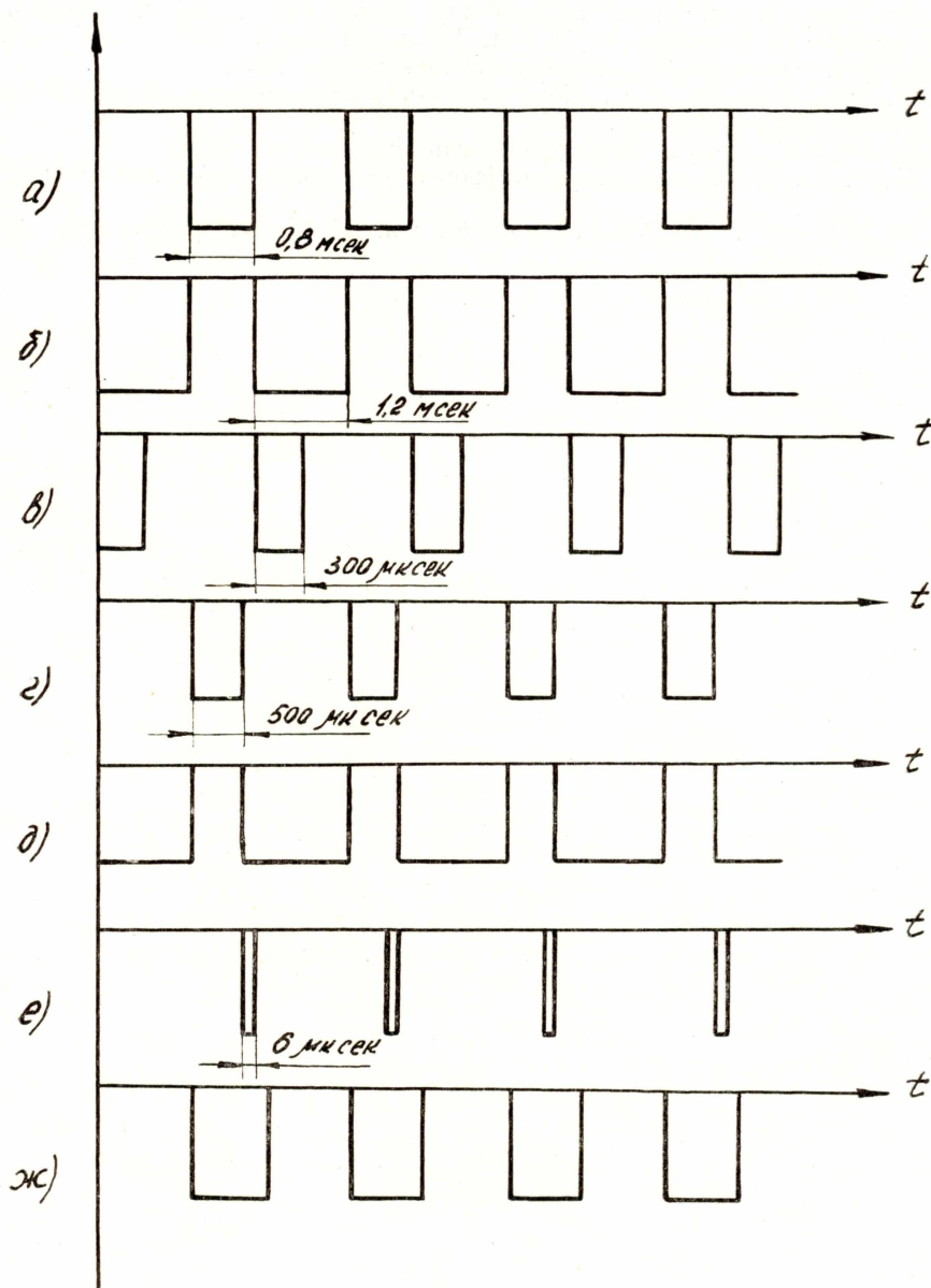
Рис. 2. Временная диаграмма работы преобразователя «Код — аналог» с ЭЦВМ.
