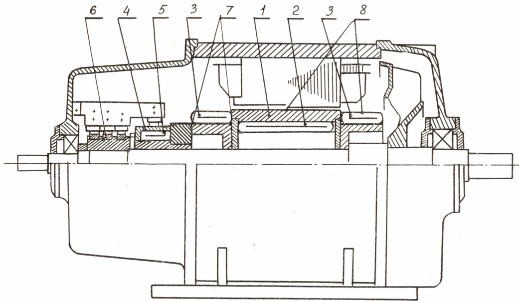
Рис. 1. Макет двигателя.
