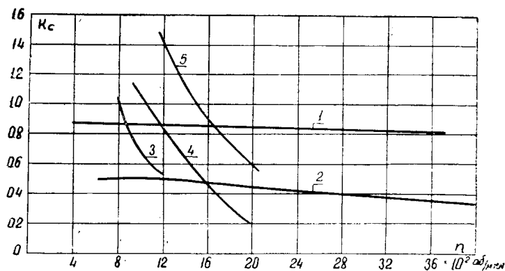
Рис. 3. Зависимость k_c от скорости вращения. 1 — ПЗ2, 2 i_a = 6a , ВМК; 2 — П40, 2 i_a = 13a , ВМК; 3 — ПЗ2, 2 i_a = 6a , ОК; 4 — П40, 2 i_a = 13a , ОК; 5 — П40, 2 i_a = 8a , ОК
