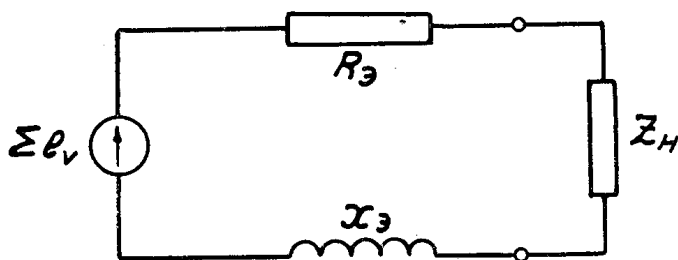
Рис. 5. Схема для расчета пульсации тока и напряжения
