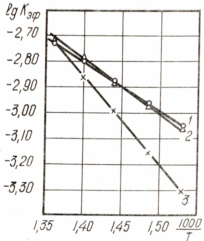
Рис. 2. Зависимость \lg K_{эф} от 1/T для процесса выделения летучих продуктов. 1. Уголь бертинированный при 200°C. 2. Уголь бертинированный при 250°C. 3. Уголь бертинированный при 300°C.
