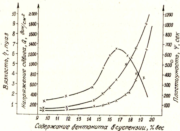
Рис. 2. Влияние концентрации бентонитовой суспензии на реологические свойства.
