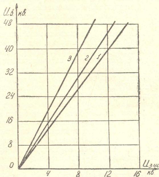
Рис. 1. Зависимости U_{з.щ} = f(U_{в.и}) 1 — R_{з.щ} = 3,3 \text{ Ом} 2 — R_{з.щ} = 2,5 \text{ Ом} 3 — R_{з.щ} = 1,5 \text{ Ом}
