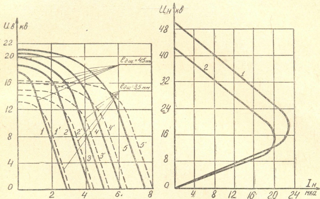
Рис. 2. Зависимости U_b = f(I_n) для дополнительного ротора: 1,1' — U_b = 18 кв; 2,2' — U_b = 24 кв; 3,3' — U_b = 30 кв; 4,4' — U_b = 34 кв; 5,5' — U_b = 40 кв
