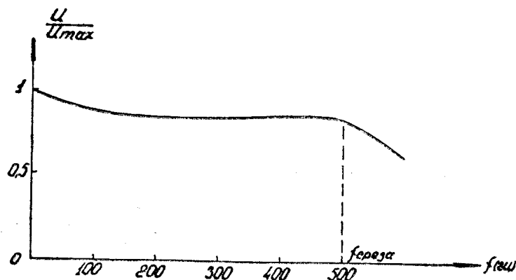
Рис. 2. Частотная характеристика фильтра низких частот
