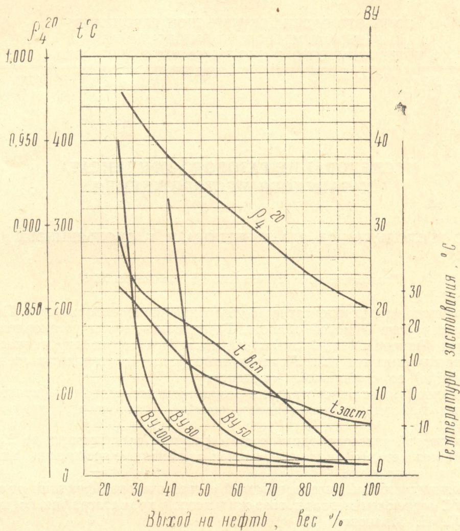
Рис. 3. Характеристика остатков самотлорской нефти.
