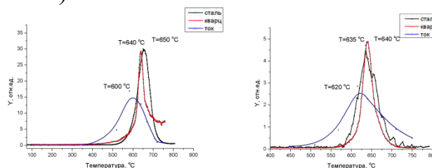
Рис. 4. Выход изотопов водорода (а- H_2 , б- D_2 ) из Ti в режиме линейного нагрева 1 – Нагрев кварцевой коаксиальной печью вакуумной ячейке из нержавеющей стали:
