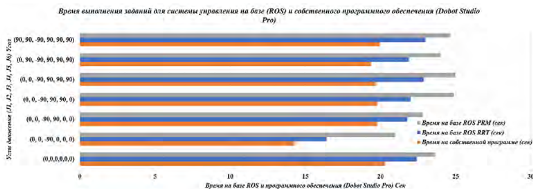
Рис. 4. Сравнение времени выполнения задач управления Dobot CR3 в ROS и Dobot Studio Pro
