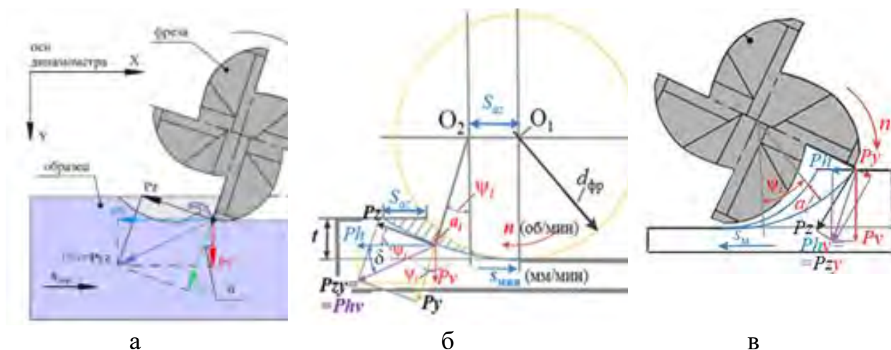
Рис. 2. Схемы действия сил: а – при врезании зуба фрезы при встречном фрезеровании, б – в промежуточном положении зуба при встречном фрезеровании, в – при врезании зуба фрезы при попутном фрезеровании
