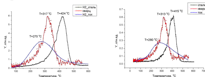
Рис. 1. Выход изотопов водорода (a- H_2 , b- D_2 ) из Ni в режиме линейного нагрева 1 – Нагрев кварцевой коаксиальной печью вакуумной ячейке из нержавеющей стали:
