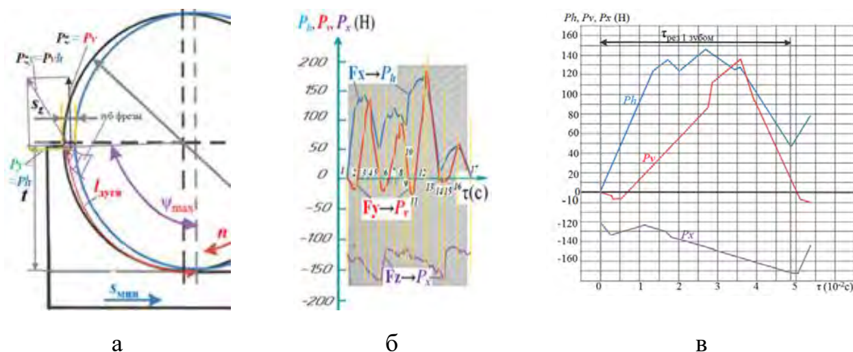
Рис. 4. Направление технологических составляющих силы резания ( P_{z_{\text{max}}} \approx P_{v_{\text{max}}} ; P_{y_{\text{max}}} \approx P_{h_{\text{max}}} ) перед выходом зуба из контакта с заготовкой (а); графики изменения сил при повороте острой фрезы на один оборот при встречном фрезеровании четырехзубной неизношенной фрезой \varnothing d = 8 мм, t = 3,8 мм, B = 2 мм, n = 500 об/мин, s_{\text{м}} = 28 мм/мин, 40Х13 (образец № 1 АТ) – твердый сплав ВК8 (б); графики изменения составляющих силы фрезерования при резании одним зубом (в)
