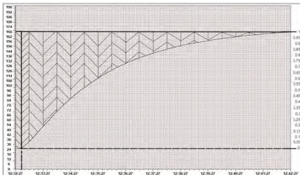
Рис. 4. Определение T объекта методом Симою
