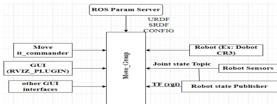
Рис. 1. Архитектура системы управления роботом на базе ROS
