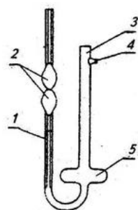
Рис. 1. Вискозиметр Освальда–Пинкевича: 1 – капиллярная трубка; 2 – калиброванные расширения; 3 – широкая трубка; 4 – отводной отросток; 5 – емкость для нагревания.
