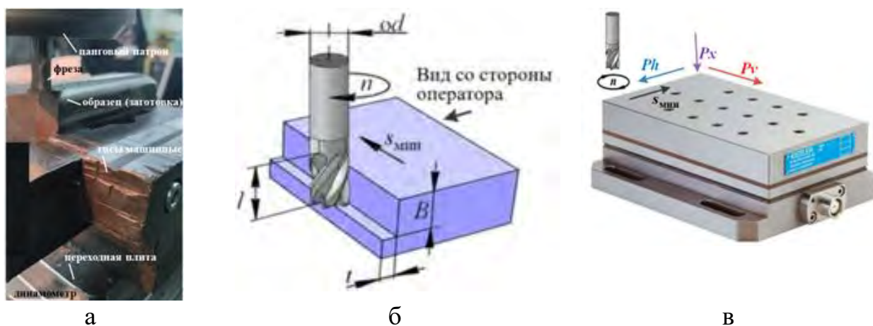
Рис. 1. Фрезирование образца на вертикально-фрезерном станке ФУ251: а – общий вид, б – схема фрезирования, в – направления сил, измеряемых динамометром Kisler, при встречном фрезировании образца
