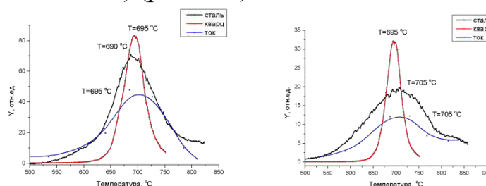
Рис. 5. Выход изотопов водорода (а- H_2 , б- D_2 ) из Zr (Э110) в режиме линейного нагрева 1 – Нагрев кварцевой коаксиальной печью вакуумной ячейки из нержавеющей стали:
