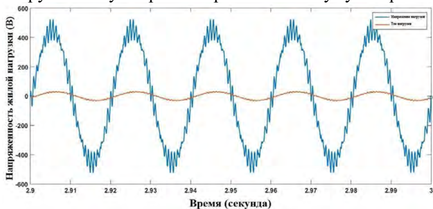
Рис. 16. Напряжение и ток бытовой нагрузки в режиме работы от аккумулятора
