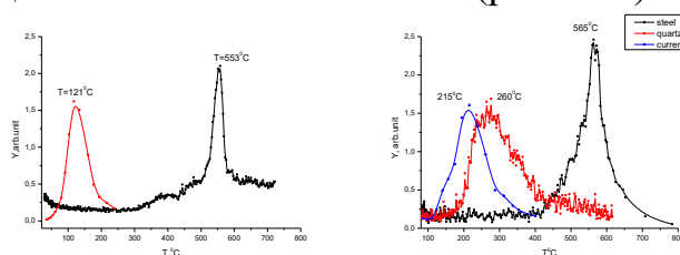
Рис. 3. Выход изотопов водорода (a-H 2 , b-D 2 ) из Pt в режиме линейного нагрева 1 – Нагрев кварцевой коаксиальной пещью в вакуумной ячейке из нержавеющей стали: T_{max}(H_2)=555\text{ }^{\circ}\text{C} , T_{max}(D_2)=565\text{ }^{\circ}\text{C}
