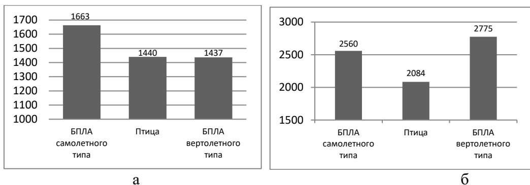
Рис. 2. Количество объектов по классам в датасетах: а – датасет с изображениями ЛО малых размеров; б – датасет с изображениями разномасштабных ЛО
