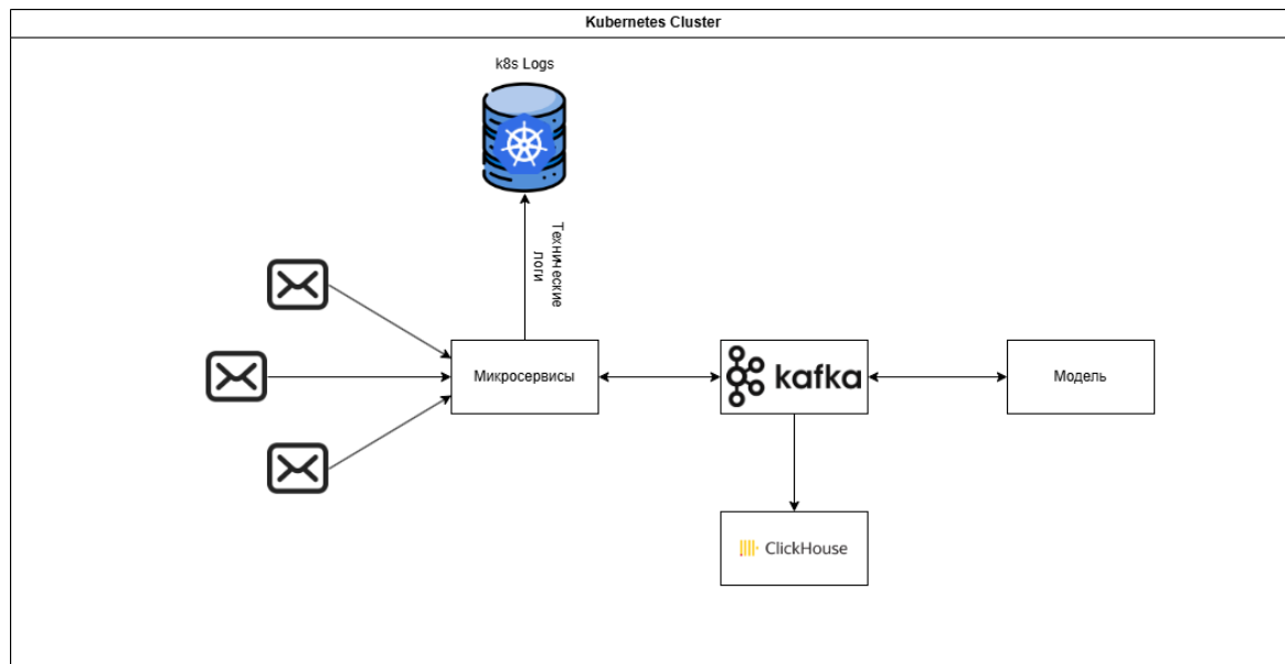
Рис. 2. Архитектура системы с использованием Kubernetes
