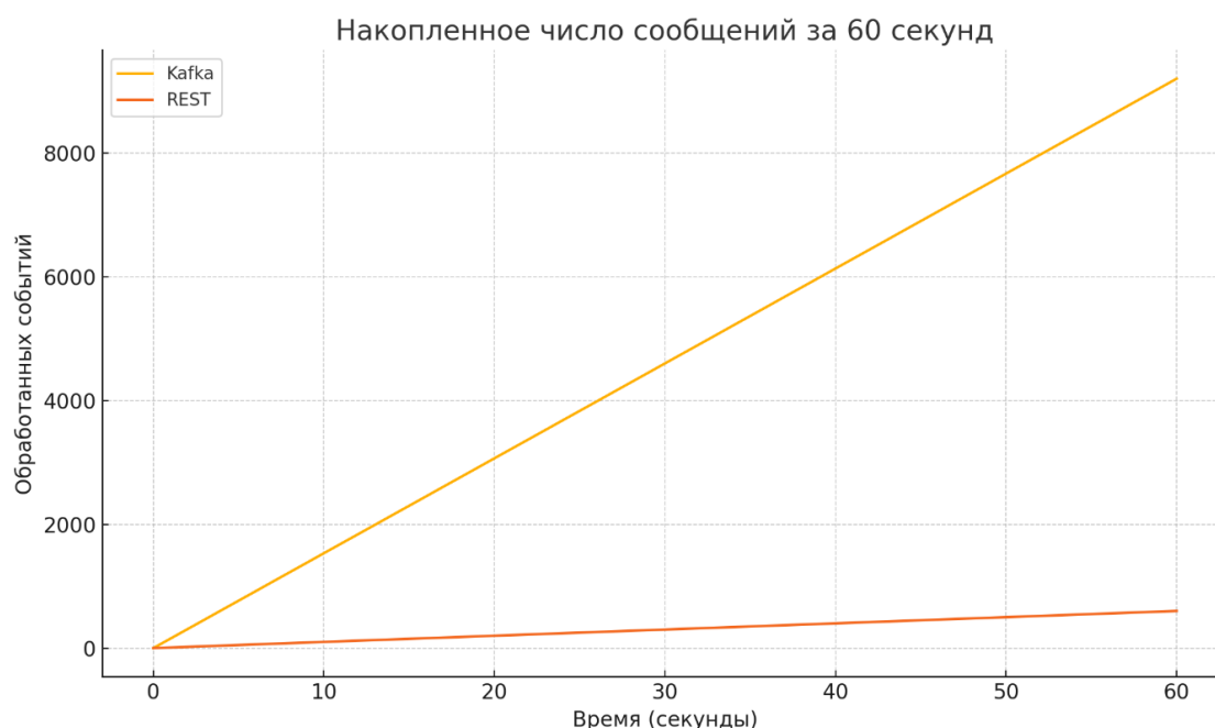
Рис. 4. График сравнения обработки запросов с использованием REST и Kafka
