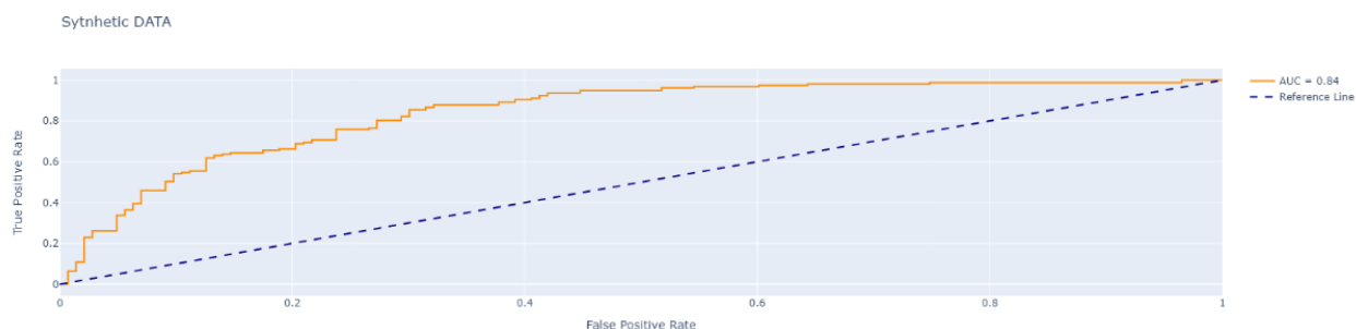
Рис. 2. ROC-кривые синтетического датасета
