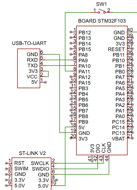
Рис. 2. Схема подключений Fig. 2. Connection scheme
