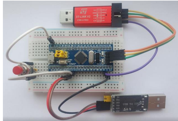
Рис. 3. Фото собранной схемы
