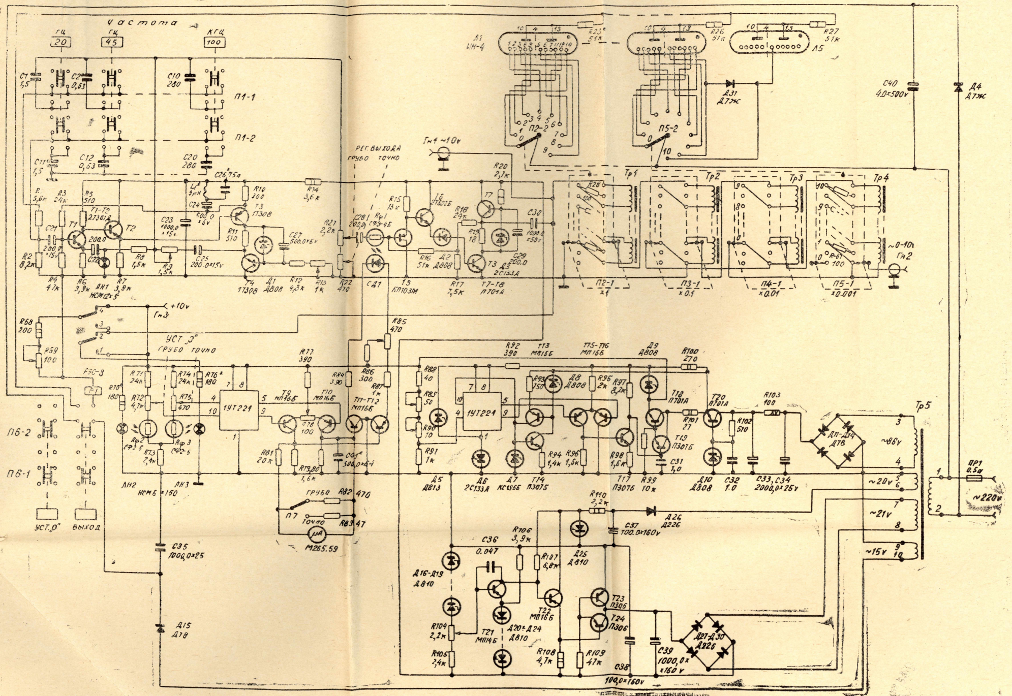
Рис. 2. Принципиальная схема ГК-10
