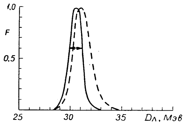
Рис. 4. Нормированная функция правдоподобия в зависимости от D_\Lambda при \rho=0 — сплошная кривая и при \rho = 1/2 — пунктирная кривая. Отрезок внутри кривой определяет интервал, соответствующий одному стандартному отклонению.
