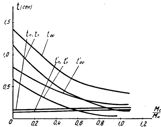
Рис. 2. Зависимости t_n; t_T; t_{oc} от M_c при значе-
