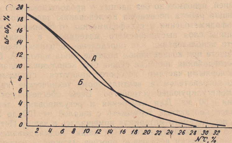
Рис. 1. Обобщенные кривые сушки. А — для сульфодиметоксина; Б — для сульфодимезина
