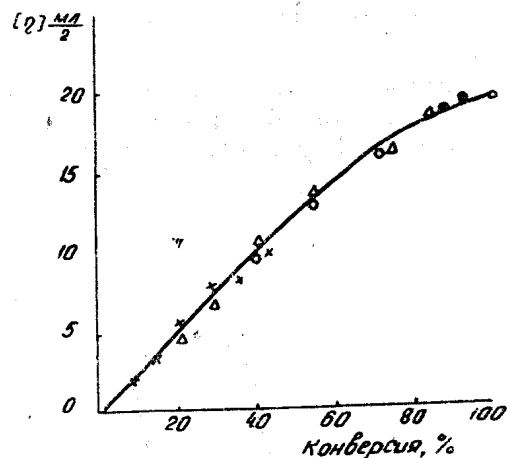
Рис. 8. Зависимость характеристической вязкости поли-3-хлор-9-винилкарбазола от конверсии мономера при различных концентрациях хлорного олова: X — 7,7 · 10 -6 моль/л;
