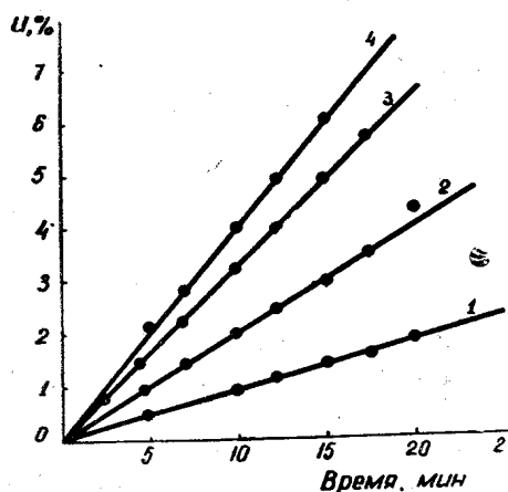
Рис. 2. Кинетика полимеризации 3-хлор-9-винилкарбазола в растворе бензола при 60^\circ С. Концентрации: мономера — 0,78 моль/л; инициатора ДАК: 1 — 9,00 \cdot 10^{-4} моль/л; 2 — 4,65 \cdot 10^{-3} моль/л; 3 — 9,15 \cdot 10^{-3} моль/л; 4 — 1,64 \cdot 10^{-2} моль/л
