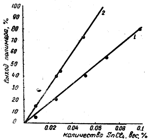
Рис. 7. Зависимость выхода поли-3-хлор-9-винилкарбазола от концентрации хлорного олова при 25° С.
