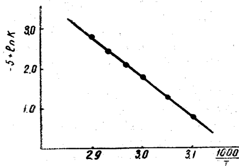
Рис. 4. Зависимость \ln K от 1/T для полимеризации 3-хлор-9-винилкарбазола. Концентрация ДАК — 9,15 \cdot 10^{-3} моль/л
