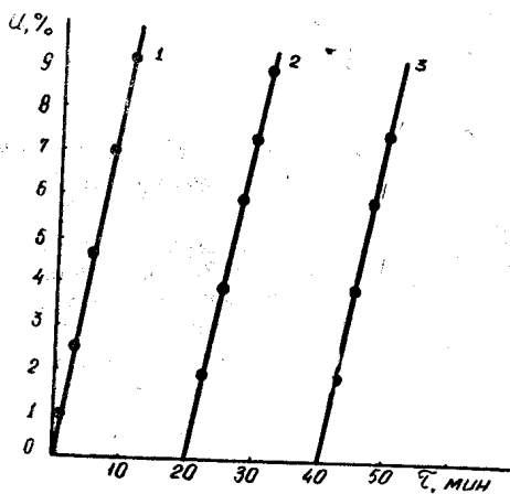
Рис. 5. Кинетика ингибированной полимеризации 3-хлор-9-винилкарбазола в присутствии бензохинона при 75° С в растворе бензола. Концентрация бензохинона: 1 — без ингибитора; 2 — 1,20 \cdot 10^{-3} моль/л; 3 — 2,40 \cdot 10^{-3} моль/л
