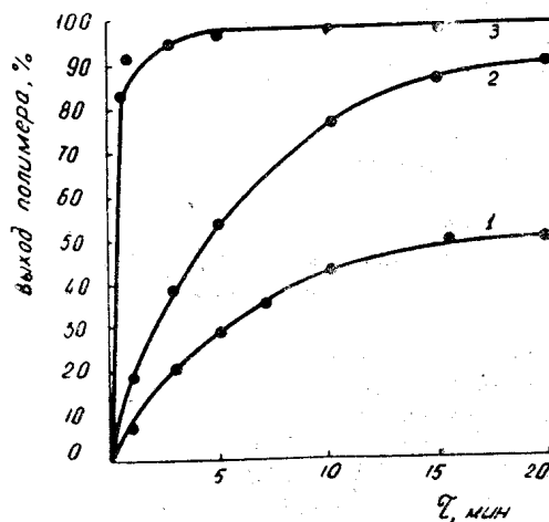
Рис. 6. Полимеризация 3-хлор-9-винилкарбазола в растворе бензола при 25° С в присутствии хлорного олова. Концентрация мономера — 0,088 моль/л. Концентрация хлорного олова: 1 — 7,70 \cdot 10^{-6} моль/л; 2 — 19,25 \cdot 10^{-6} моль/л; 3 — растворитель ДХЭ: концентрация хлорного олова 19,25 \cdot 10^{-6} моль/л
