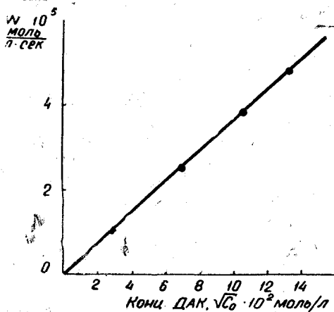
Рис. 3. Зависимость скорости полимеризации 3-хлор-9-винилкарбазола от концентрации ДАК при 60° С
