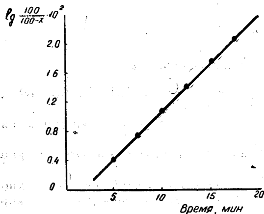
Рис. 1. Зависимость \lg \frac{100}{100-x} от времени при инициированной полимеризации 9-ВК при 60^\circ С. x — конверсия, %
