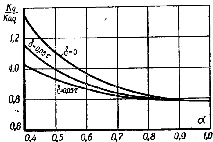
Рис. 2. Кривые для определения отношения \frac{k_q}{k_{aq}} явнополюсных машин при \frac{\delta_{\max}}{\delta} = 1,0 .
