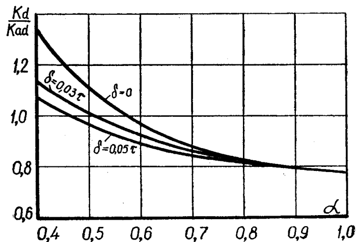
Рис. 1. Кривые для определения отношения \frac{k_d}{k_{ad}} явнополюсных машин при \frac{\delta_{\max}}{\delta} = 1,0 .
