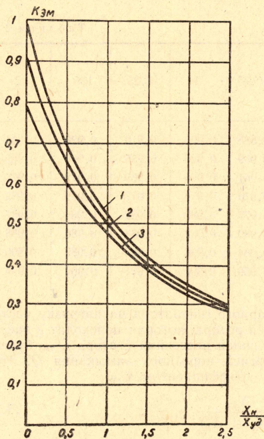
Рис. 1 Зависимость коэффициента \kappa_{эм} от отношения \frac{X_H}{X_{уд}} при 1 — r_H = 0 ; 2 — r_H = r_r ; 3 — r_H = 3r_r .
