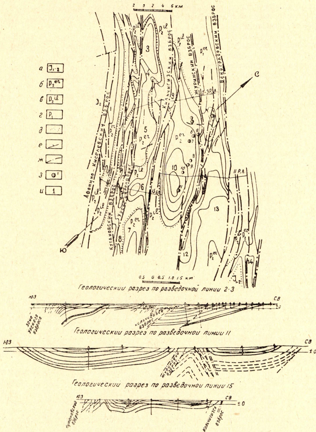
Рис. 1. Схематическая геологическая карта Ленинского района Кузбасса (трест Кузбассуглегеология 1961): а — конгломератовая свита; б — еруановская свита; в — ильинская свита; г — кузнецкая свита; д — границы свит; е — выходы пластов угля под наносы; ж — дизъюнктивы; з — стволы шахт: 1 — им. Е. Ярославского, 2 — «Журилки 3», 3 — им. Е. Ярославского (старой), 4 — им. С. М. Кирова, 5 — «Новой», 6 — «Комсомолец», 7 — «7 Ноября», 8 — «Полысаевской-1», 9 — «Полысаевской-Северной», 10 — «Полысаевской-11», 11 — «Полысаевской-III»; и — номера, указывающие на карте следующие структуры: 1 — Устюжанинская синклиналь, 2 — Новороссийская антиклиналь, 3 — Касьминская синклиналь, 4 — Мусохрановская антиклиналь, 5 — Никитинская синклиналь, 6 — Калиновская антиклиналь, 7 — Беловская синклиналь, 8 — Бабанакловская антиклиналь, 9 — Зайнская синклиналь, 10 — Ленинская синклиналь, 11 — Егоровская синклиналь, 12 — Мохово-Пестеревская антиклиналь, 13 — Красноярская синклиналь, 14 — Урупская антиклиналь.
