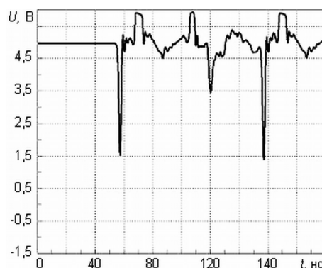
Рис. 5. Разновидности искажения сигналов в проводниках: а) искажение фронта сигнала из-за эффекта отражений, б) искажение постоянного сигнала из-за перекрестных помех
