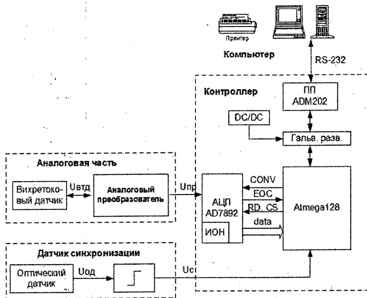
Рис. 2. Функциональная схема
