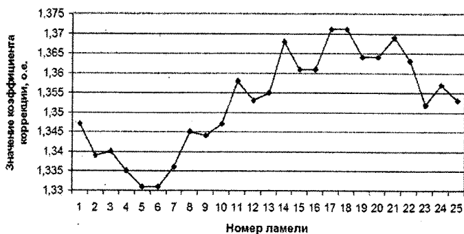
Рис. 4. Пример кривой изменения значений коэффициентов коррекции
