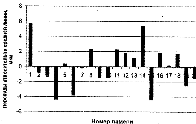
Рис. 6. Пример изменения значений перепадов между ламелями вдоль окружности коллектора
