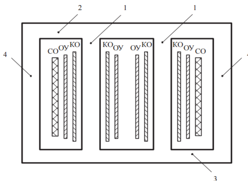
Рисунок 2.1 – Разрез магнитной системы фазы УШР 220 кВ:
