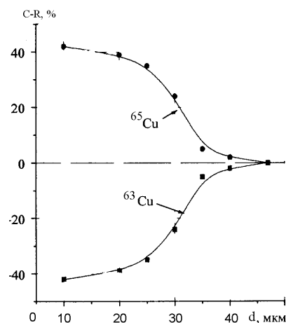
Рис. 5. Профиль отклонений изотопного состава меди в никеле от природного после диффузии в условиях ползуемости
