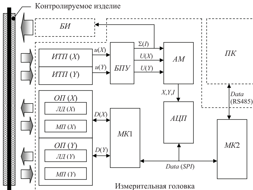
Рис. 4. Функциональная схема измерителя эксцентриситета и диаметра электрического кабеля
