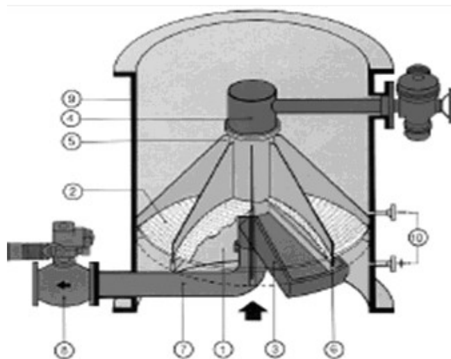
Рисунок 5 - Схема фильтра предочистки [1]
