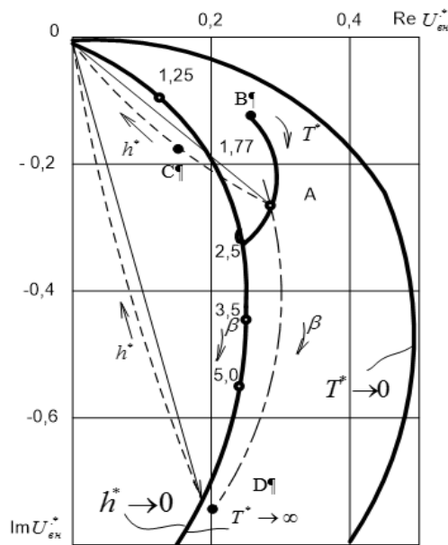
Рисунок 1.12 – Годограф U_{вн}^* при двухчастотном контроле
