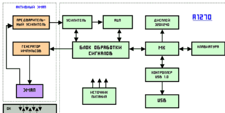
Рисунок 1.8 – Функциональная схема ЭМА толщиномера А1270
