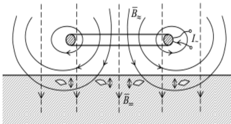
Рисунок 1.5 – Возбуждение акустических волн за счет магнитоупругого взаимодействия
