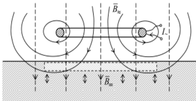
Рисунок 1.6 – Возбуждение акустических волн за счет магнитного взаимодействия
