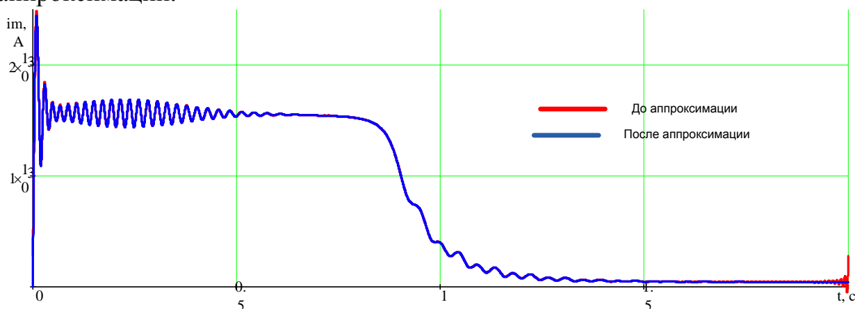
Рисунок 20 – Графики модуля результирующего вектора тока статора при пуске АД на холостом ходу без повреждений ротора до и после аппроксимации
