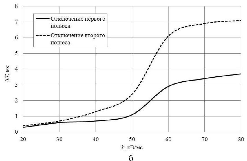
Рисунок 6 – Допустимые разбросы времени размыкания полюсов синхронного выключателя в зависимости от мощности трансформатора (а) и скорости восстановления электрической прочности межконтактного промежутка (б)
