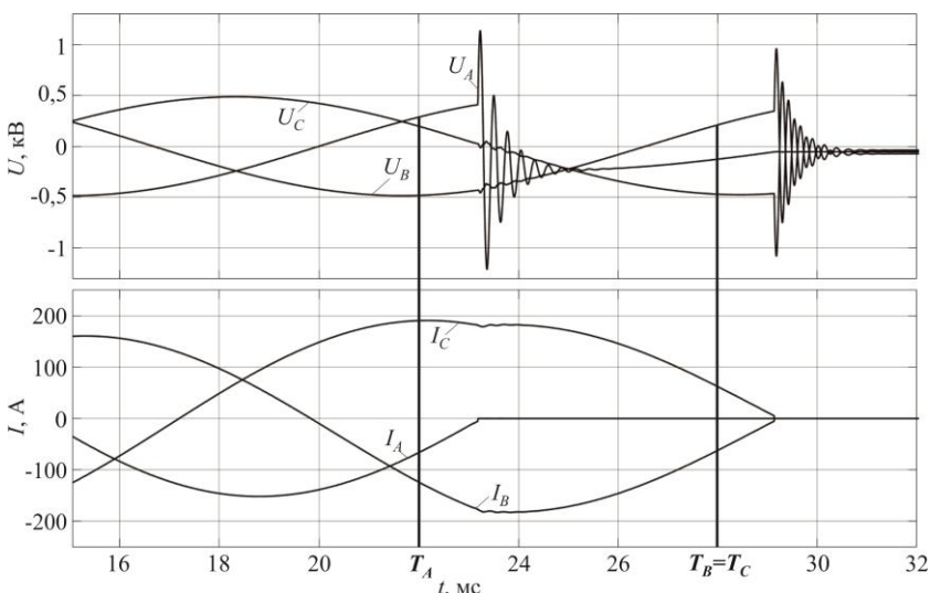
Рисунок 9 – Управляемое отключение пускового тока электродвигателя ( P_{дв} = 200 кВт, L = 25 м) по алгоритму A-BC
