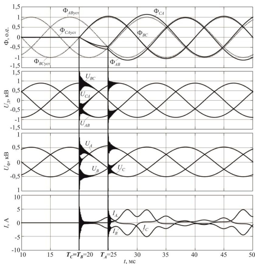
Рисунок 7 – Управляемое включение трансформатора 1000 кВА с соединением первичной обмотки в треугольник по алгоритму CB-A : \Phi – магнитный поток в сердечнике трансформатора; U_{л} , U_{ф} – линейное и фазное напряжение в электрической сети до выключателя; I – ток трансформатора
