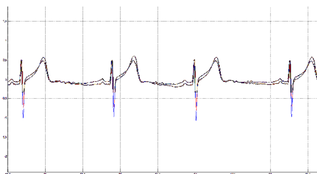
Рис. 5. Результаты сравнения емкостных сенсоров и хлорсеребряных электродов
