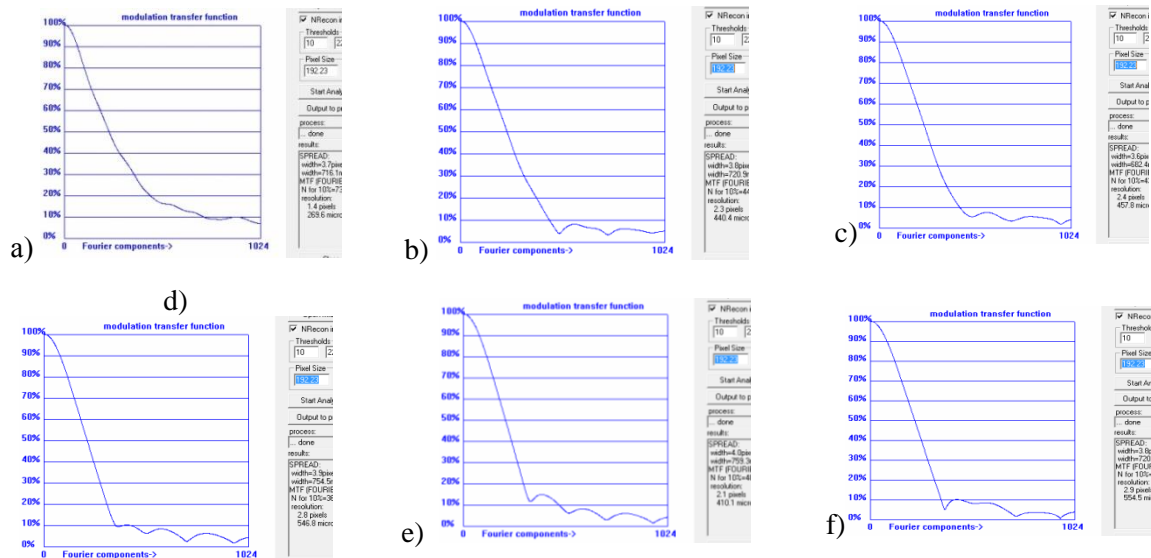
Figure 4. MTF: a) – 1 MeV; b) – 1,5 MeV; c) – 2 MeV; d) – 3 MeV; e) – 3,5 MeV; f) – 4 MeV.
