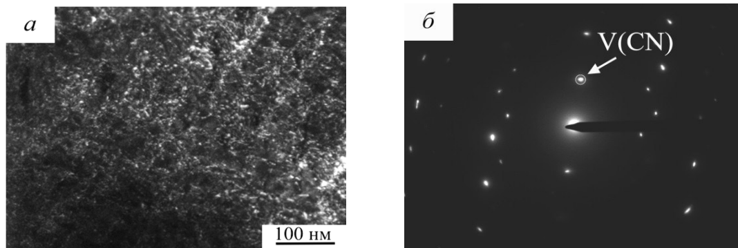
Рис. 1. Темнопольное изображение в рефлексе карбонитрида V(C, N) (а) и соответствующая микродифракционная картина (б) стали ЭК-181 после ВТМО без отпуска с деформацией в аустенитной области \epsilon \approx 30\%
