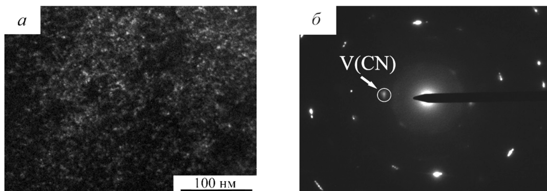
Рис. 2. Темнопольное изображение в рефлексе карбонитрида V(C, N) (а) и соответствующая микродифракционная картина (б) стали ЭК-181 после ВТМО с отпуском и деформацией в аустенитной области \epsilon \approx 60\%
