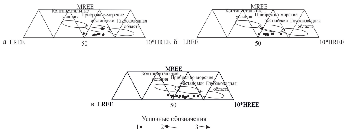
Рис. 2 Диаграмма LREE–MREE– 10^*HREE для разделения морских и континентальных осадков [3]: а – цикл 1 пласта P_1 , б – цикл 2 пласта P_1 , в – пласт P_2 . Условные обозначения: 1 – фигуративные точки пород; 2 – регрессивный режим; 3 – трансгрессивный режим
