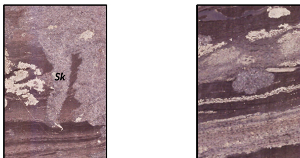
Рис. 2. Увеличенные фрагменты. Слева – ход Skolithos , справа – канал отлива
