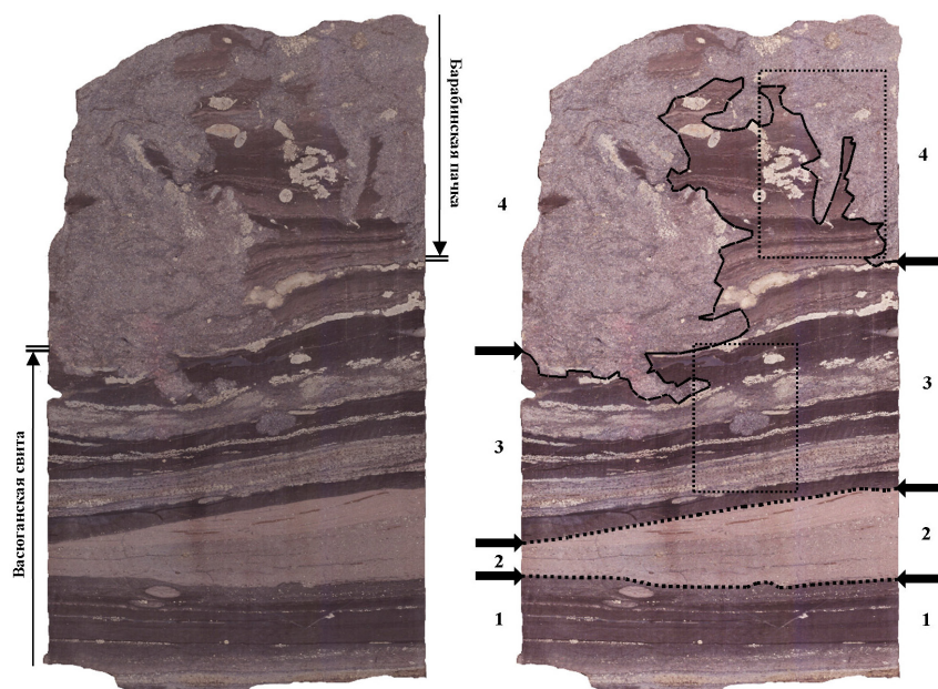
Рис. 1. Сканированное изображение образца. Слева – интервалы васюганской свиты и барабинской пачки; справа – выделение интервалов (контрастность +20%) и увеличенных фрагментов (прямоугольники) в образце
