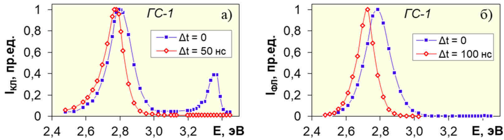
Рис. 6. Нормированные спектры время-разрешенной люминесценции образца ГС-1 при возбуждении СЭП с H = 0,01 \text{ Дж/см}^2 (а) и N_2 -лазером с W = 2 \cdot 10^4 \text{ Вт/см}^2 (б).
