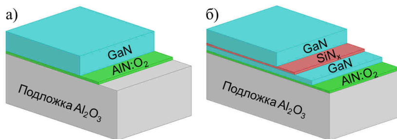
Рис. 2. Структура образцов GaN-1 (а) и GaN-2 – GaN-4 (б).
