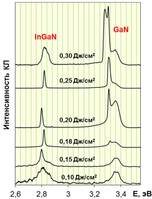
Рис. 3. Спектры КЛ образца ГС-2 при облучении СЭП с разной плотностью энергии, масштабированные таким образом, что интенсивность КЛ полосы InGaN при всех уровнях возбуждения одинакова. T = 300 К.
