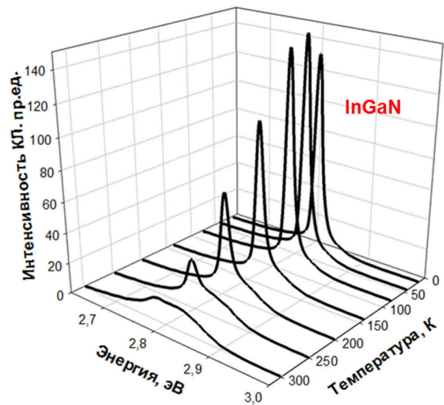
Рис. 4. Температурная зависимость спектров КЛ полосы InGaN образца ГС-1 при облучении СЭП с H = 0,056 Дж/см 2 .
