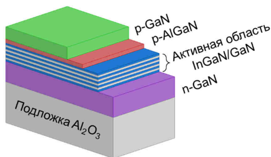
Рис. 1. Общая схема исследуемых гетероструктур ГС-1 – ГС-7.
