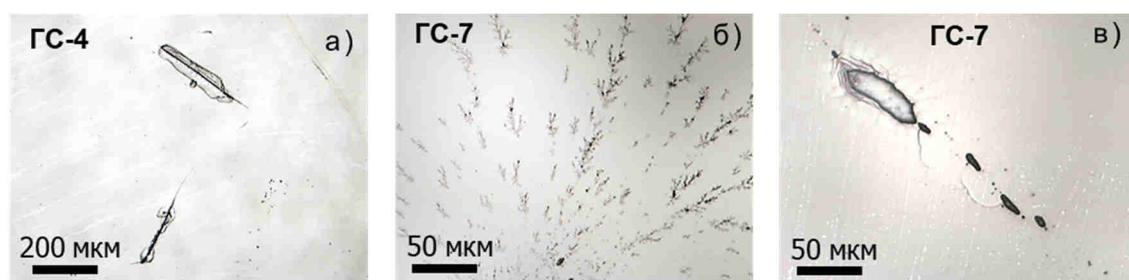
Рис. 11. Морфология разрушений в образцах ГС-4 (а) и ГС-7 (б, в) после облучения СЭП при H = 0,6 Дж/см 2 .
