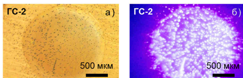
Рис. 15. Распределение микроразрушений (а) и люминесценции (б), возбуждаемой СЭП ( H = 0,25 Дж/см 2 ), по поверхности образца ГС-2. Просвечивающаяся окрестность соответствует границам диафрагмы-коллиматора ускорителя электронов.
