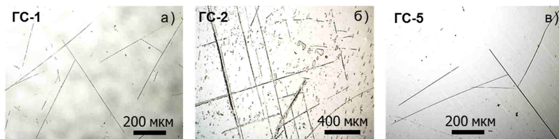
Рис. 12. Трещины, образовавшиеся в образцах ГС-1 (а), ГС-2 (б) и ГС-5 (в) после облучения СЭП при H = 1 Дж/см 2 .
