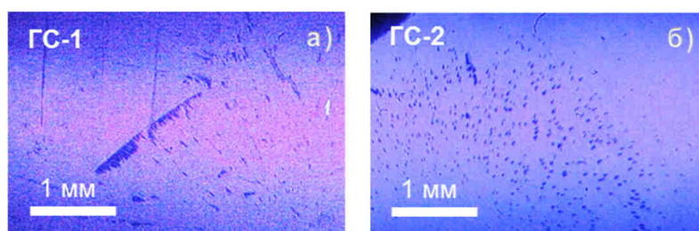
Рис. 14. Микрзоны остаточных разрушений в образцах ГС-1 (а) и ГС-2 (б) на фоне люминесценции, возбуждаемой N_2 -лазером ( W \sim 10^4 Вт/см 2 ).
