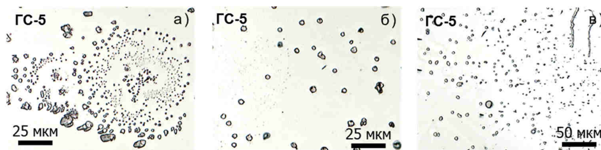
Рис. 17. Фотографии микроразрушений, образовавшихся в образце ГС-5 после многоимпульсного облучения СЭП при H = 0,25 Дж/см 2 .
