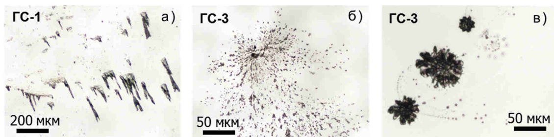
Рис. 10. Фотографии специфических микроразрушений в образцах ГС-1 (а) и ГС-3 (б, в) после многоимпульсного облучения СЭП при H = 0,25 Дж/см 2 .
