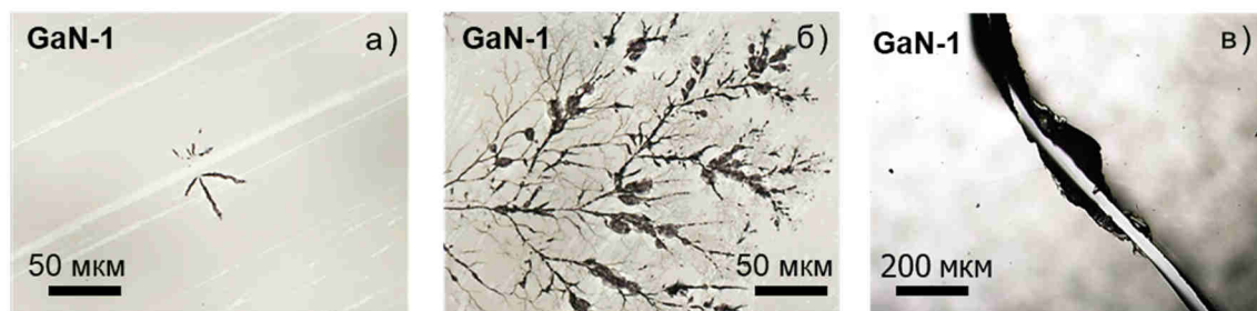
Рис. 13. Каналы электрического пробоя в образце GaN-1, сформировавшиеся под действием СЭП с H = 0,25 Дж/см 2 (а, б), и хрупкий раскол образца GaN-1 (две части образца приставлены друг к другу) при облучении СЭП с H = 0,6 Дж/см 2 (в).
