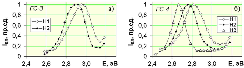
Рис. 5. Нормированные спектры КЛ InGaN-КЯ в образцах ГС-3 (а) и ГС-4 (б), измеренные при плотностях энергии СЭП: H1 = 0,25 \text{ Дж/см}^2 , H2 = 0,01 \text{ Дж/см}^2 , H3 = 0,005 \text{ Дж/см}^2 .
