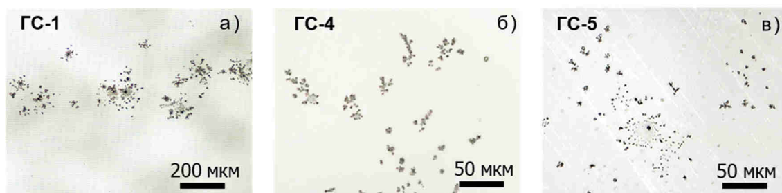
Рис. 9. Фотографии микроразрушений в образцах ГС-1 (а), ГС-4 (б), ГС-5 (в) после 10 импульсов облучения СЭП при H = 0,25 Дж/см 2 .
