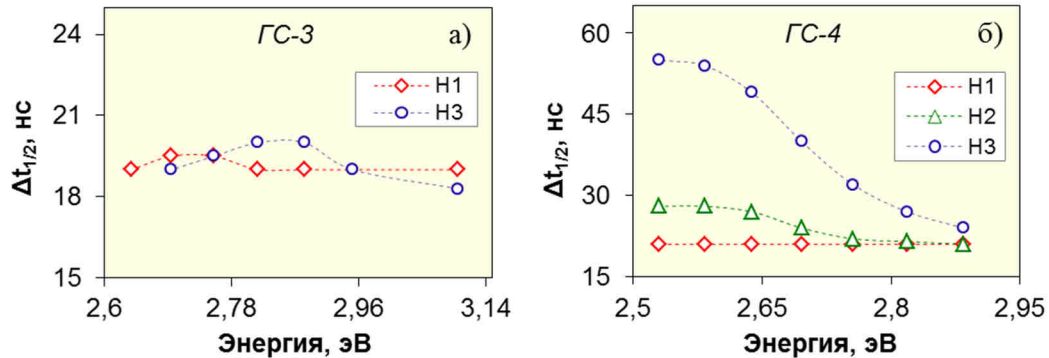
Рис. 7. Зависимость длительности импульса КЛ, измеренная на полувысоте, от энергии излучения образцов ГС-3 (а) и ГС-4 (б) при разных плотностях энергии СЭП: H1 = 0,25 \text{ Дж/см}^2 , H2 = 0,05 \text{ Дж/см}^2 , H3 = 0,01 \text{ Дж/см}^2 .
