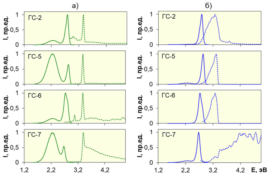
Рис. 8. Спектры люминесценции (сплошная линия), измеренные при фотовозбуждении с энергией, соответствующей максимуму спектра возбуждения (штриховая линия) желто-зеленой (а) и синей (б) ФЛ, в различных гетероструктурах.
