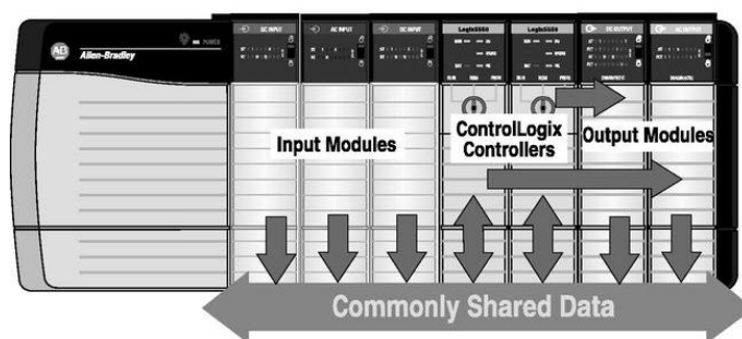
Рисунок 10 – Шасси CONTROLLOGIX CHASSIS
