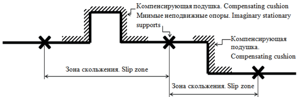
Рис. 2. Участок тепловой сети только с зонами скольжения и мнимыми неподвижными опорами Fig. 2. Section of a heat supply network with slip zones and imaginary stationary supports
