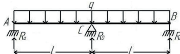
Рис. 4. Расчетная схема
