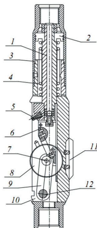
Рис. 1. Конструкция перфоратора
