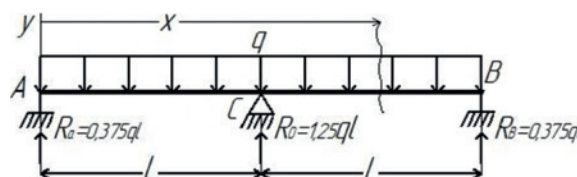
Рис. 5. Схема со значениями реакций опор
