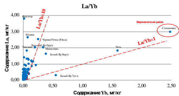
Рис. 2 La/Yb соотношение в солевых отложениях питьевых вод (накипи) Томской области
