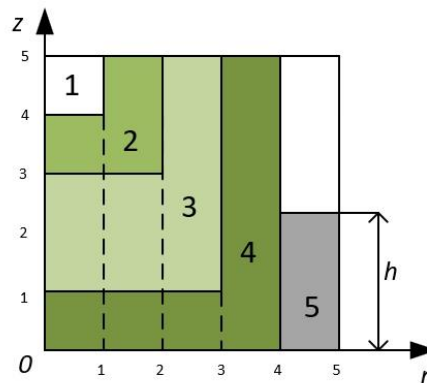
Рис. 2. Область решения задачи теплопередачи при зачеканивании датчика: 1 – спай термопары; 2 – керамический чехол; 3 – порошок оксида алюминия; 4 – внешний защитный чехол; 5 – воздушный зазор h- глубина зачеканивания
