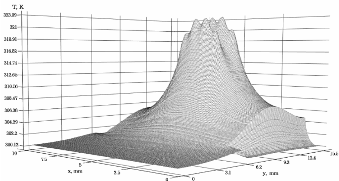
Рис. 3. Распределение температур на 3-й секунде работы ППП (транзистора)
